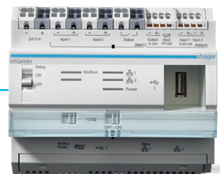
agardio.manager HTG411H Modbusfähig: – Status Schaltstellung EIN/AUS – RCD-Ausschaltvorwarnung – RCD-Schaltalarmierung
