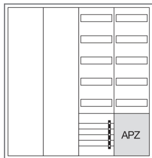
ZB34VT10APZ2
