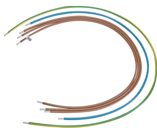
Abgangskabelbaum, univZ, 16 mm 2 , 5P, L1,2,3, N, PE=950, 950, 950, 950, 1250, H/H
