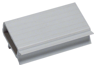
Schienenisolierprofil, univers Z, für CU 12 x 5 mm, 3 St. je 30 mm
