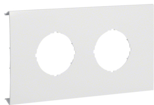
Blende 2-fach d=45mm für UP-Einsatz ohne Rahmen hfr BRH Oberteil 100mm cremeweiß
