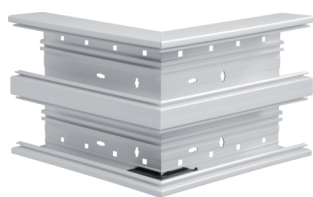
Außeneck aus Grundprofil zu BR 68x210mm Oberteil 2x80mm in lichtgrau
