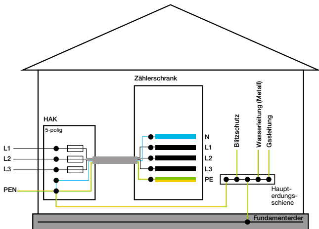
TN-System
