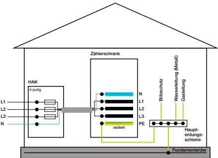
TT-System
