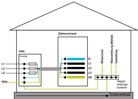
TN-System
