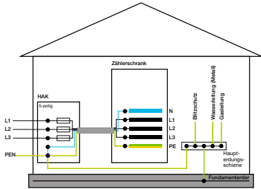
TN-System
